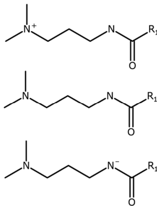
104 図 1-1 解離に係る構造式(長鎖は R として省略)
