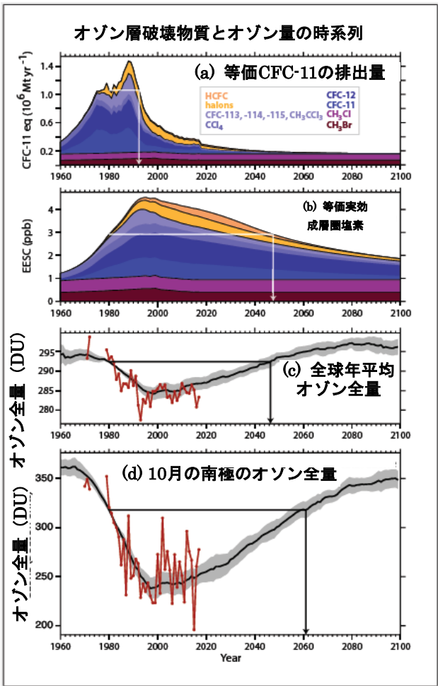
図1 オゾン層破壊物質とオゾン量の時系列
