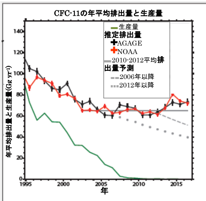
図4 CFC-11の年毎の排出量と生産量
