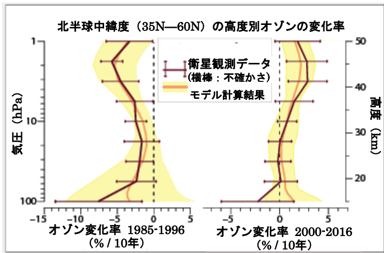
図2 成層圏オゾンの高度別の変化率 (左図：1985～1996年の10年あたりの変化率、右図：2000～2016年の10年あたりの変化率)
