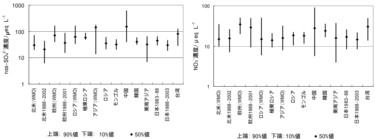
図 2 非海塩性硫酸イオン及び硝酸イオンの濃度の分布範囲
