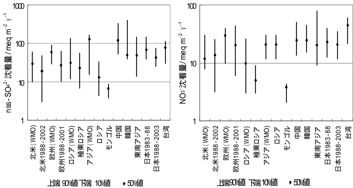
図 1 非海塩性硫酸イオン及び硝酸イオン沈着量の分布範囲
