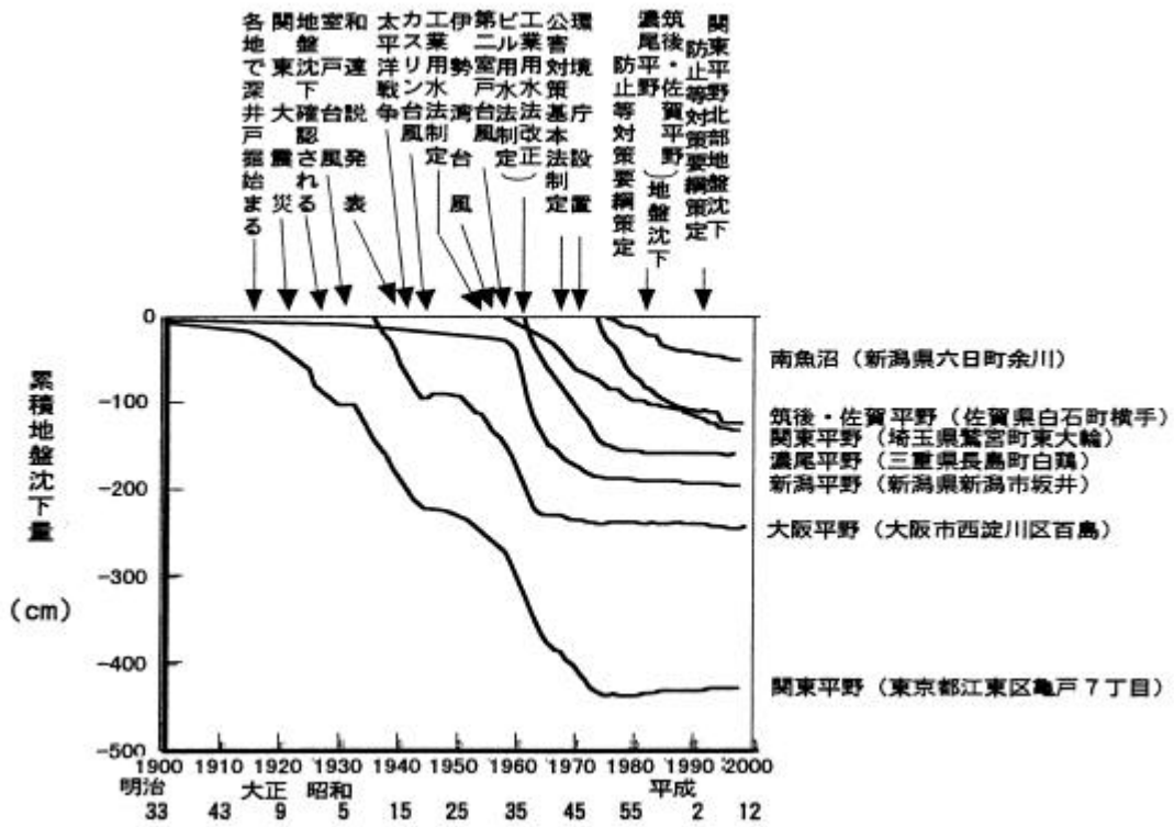
図 - 4 代表的地域の地盤沈下の経年変化
