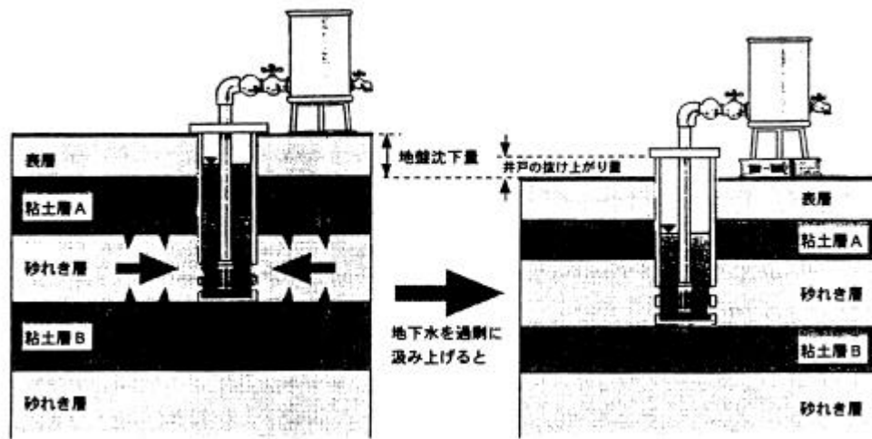
図 - 3 地盤沈下のしくみと抜け上がり現象
