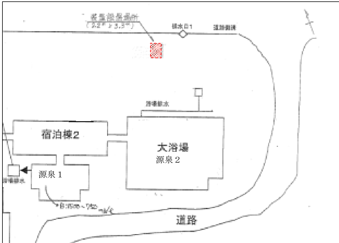
【平面配置図】
