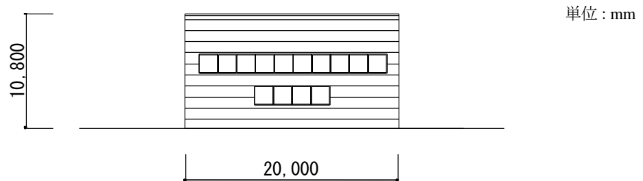
図 9 計算用工場モデル（東側立面図）
