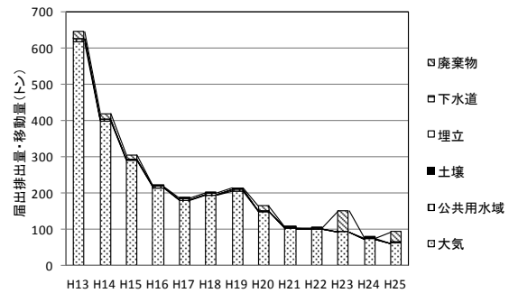
1,3-ブタジエン(351)
