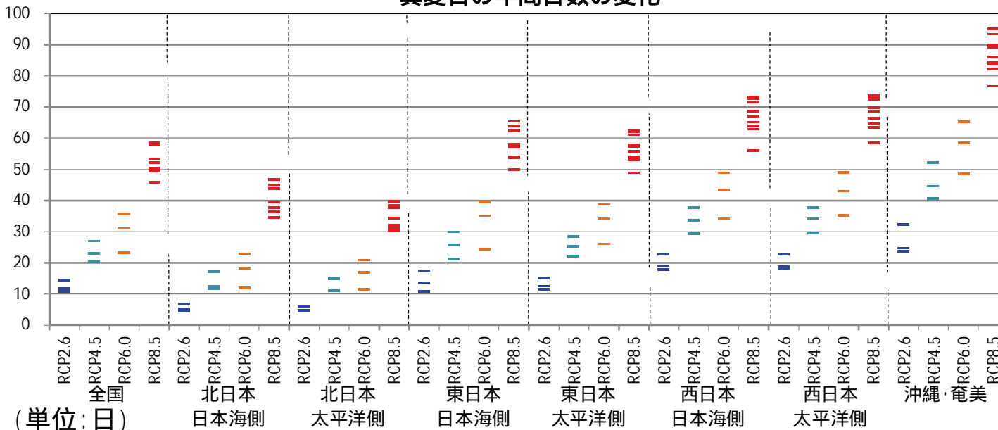
真夏日の年間日数の変化
