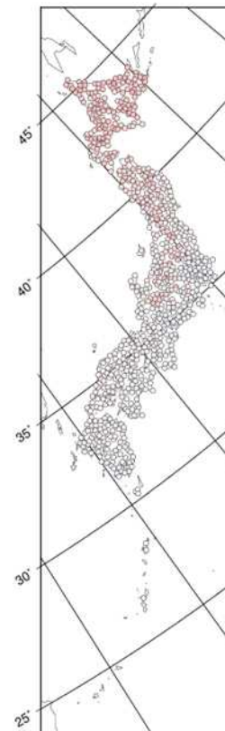
真冬日の年間日数の変化の分布(SST1,YSケースの例示)
