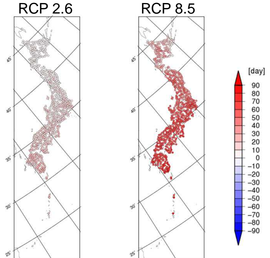
真夏日の年間日数の変化の分布(SST1, YSケースの例示)
