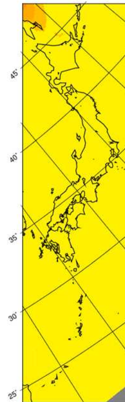
日最低気温の年平均値の変化の分布(SST1, YSケースの例示)
