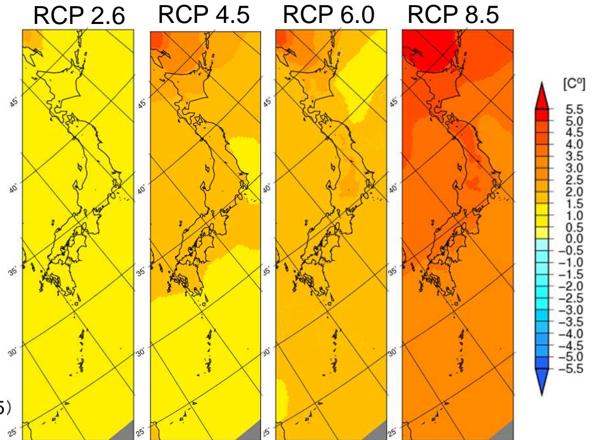
年平均気温の変化の分布(SST1, YSケースの例示)
