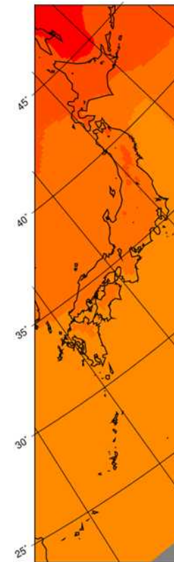
日最高気温の年平均値の変化の分布(SST1, YSケースの例示)
