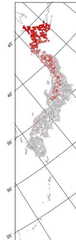
真冬日の年間日数の変化の分布(SST1,YSケースの例示)
