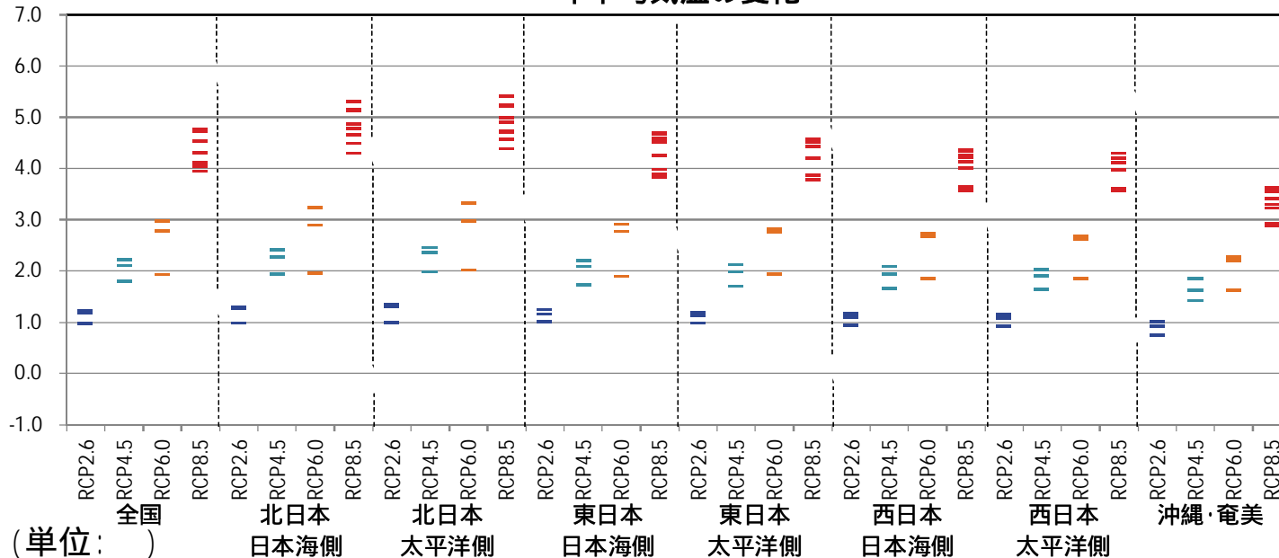
年平均気温の変化
