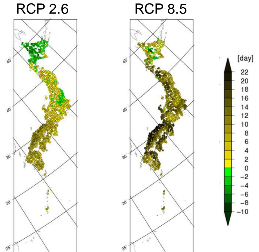
無降水日の年間日数の変化の分布(SST1, YSケースの例示)
