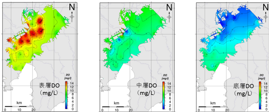
図1-1 溶存酸素量 (DO) の水平分布
