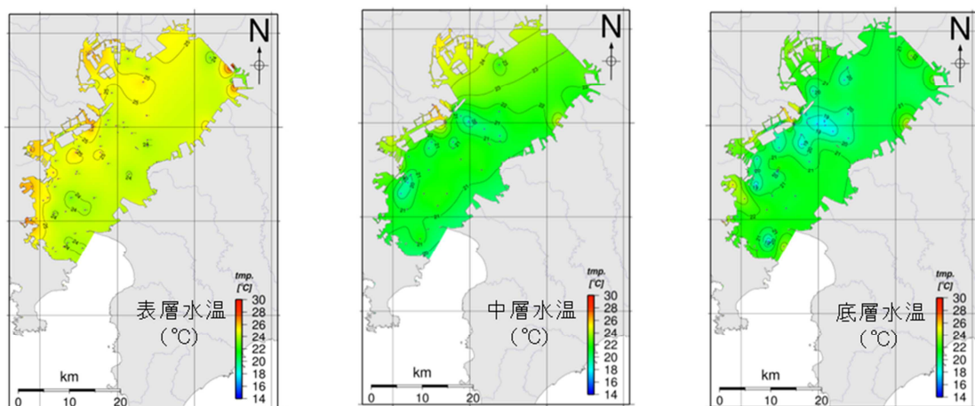
図1-2 水温の水平分布
