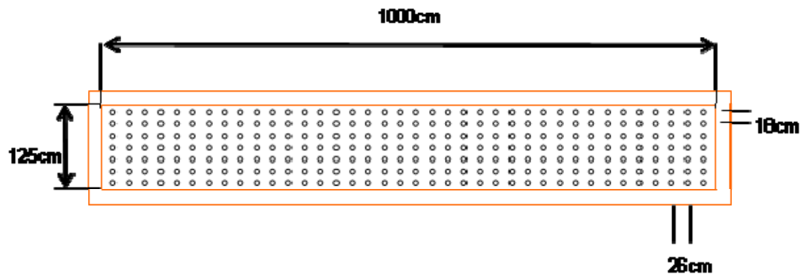
図5 枠水田の栽植計画
