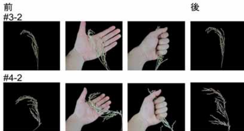
図 4 . 脱粒性
