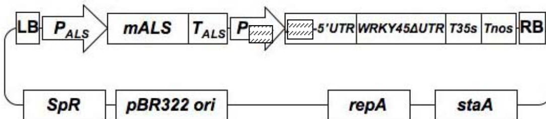
図1 本遺伝子組換えイネ作出に用いた形質転換用プラスミド(バイナリーベクター)の構造 トータルサイズ 11.3 kb
