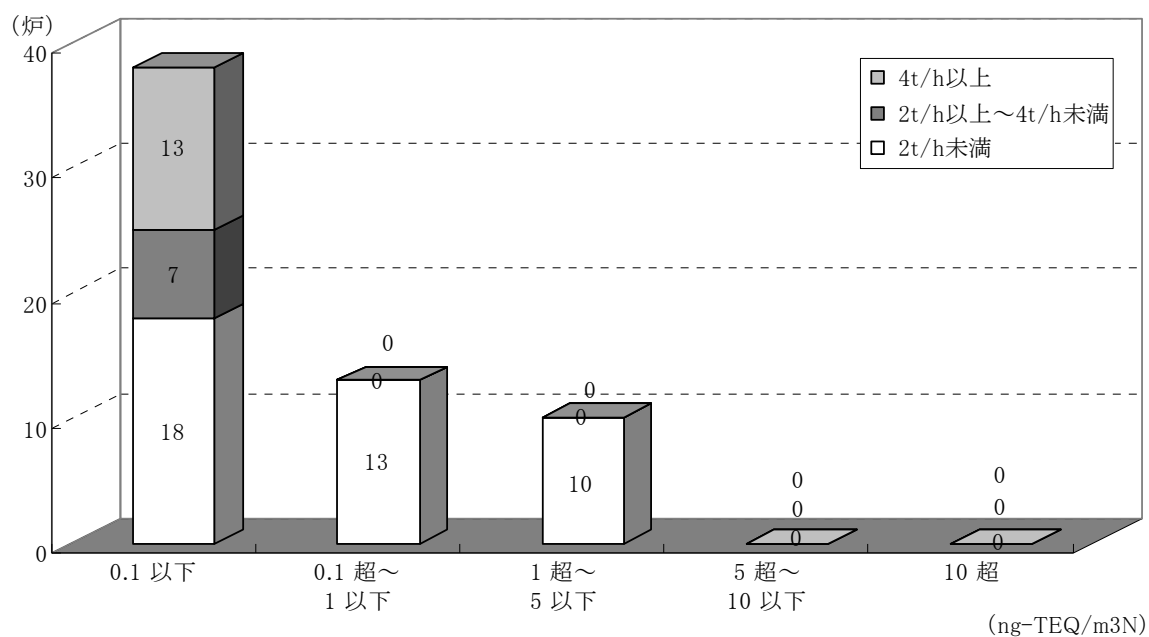
一般廃棄物焼却施設（事業者設置）の排ガス中のダイオキシン類濃度の分布
