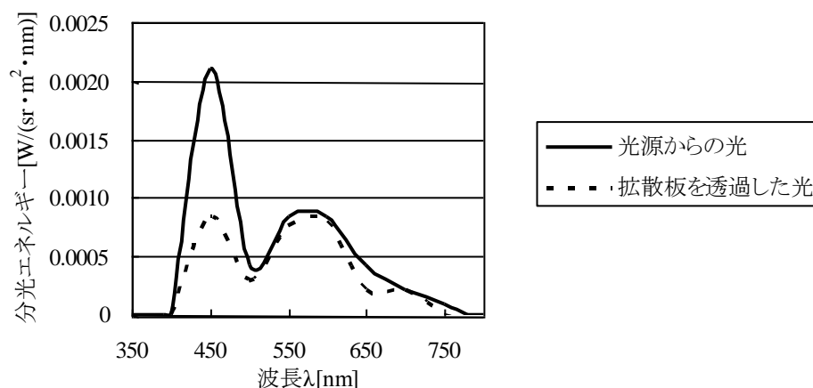
図 4 分光分布のイメージ
