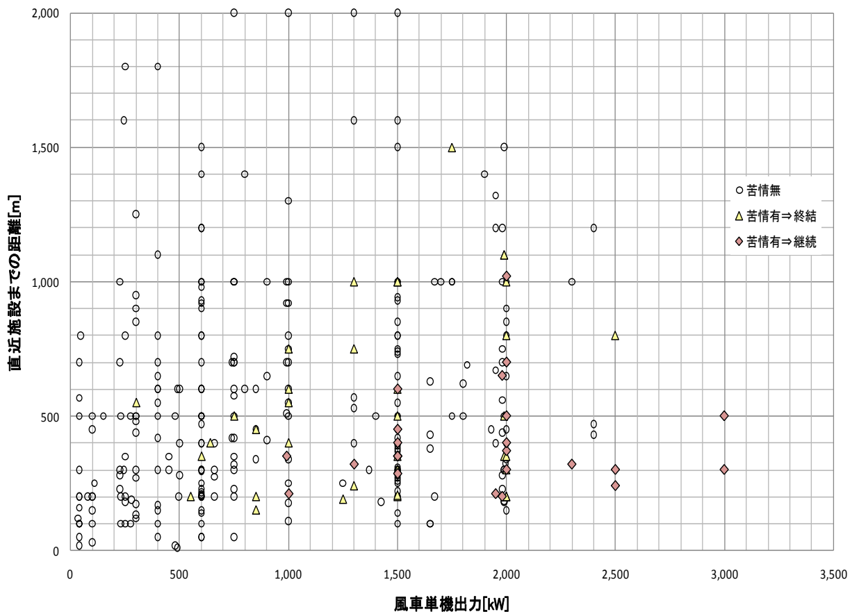
図-10 風車単機出力と直近施設までの距離
