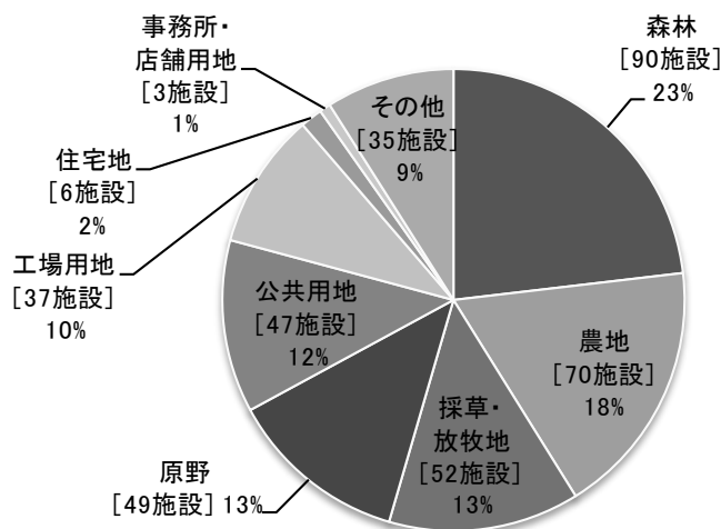
図-6 周辺の土地利用
