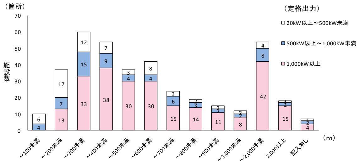
図-9 直近の住宅等までの水平距離
