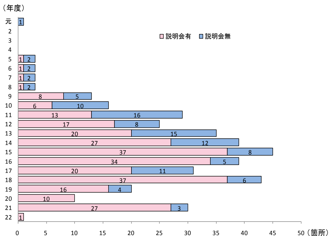
図－8 稼働年度別の住民説明会開催状況
