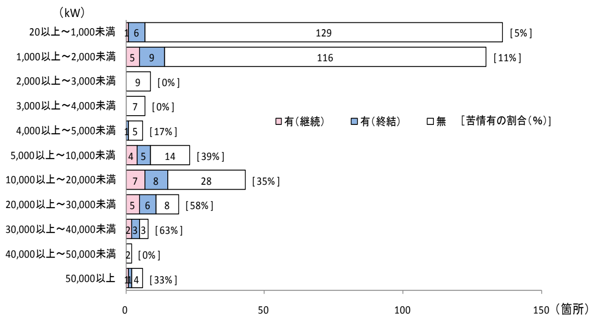
図－5 総出力別の施設箇所数
