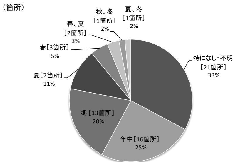
図-12 騒音・低周波音に関する苦情等が生じる季節
