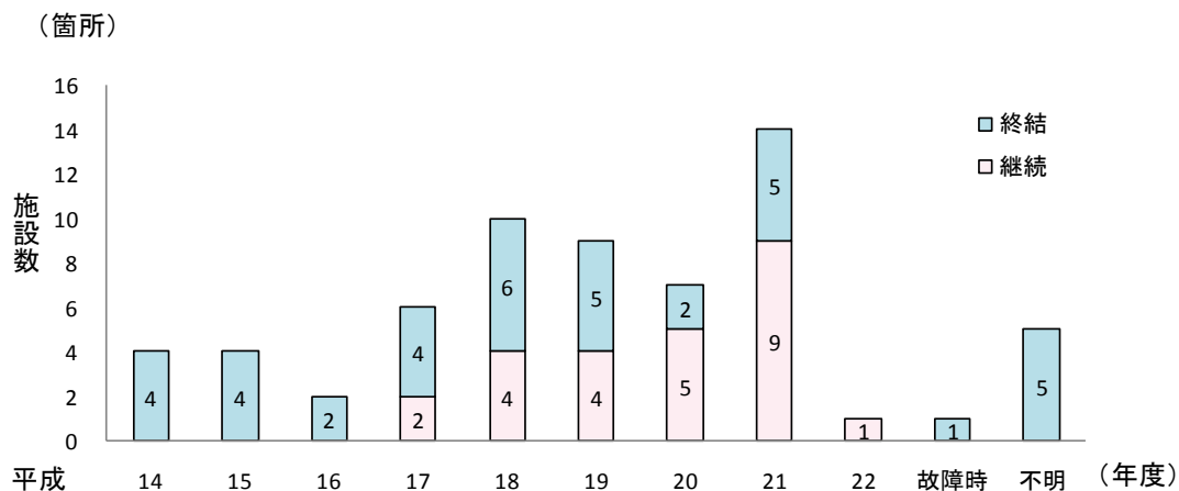
図-13 苦情等が初めて寄せられた時期
