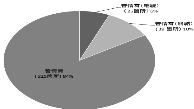
図－1 騒音・低周波音に関する苦情等の有無
