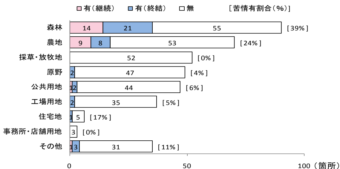
図-7 土地利用別の苦情等発生状況
