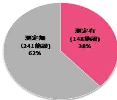
図-14 騒音・低周波音の測定の有無
