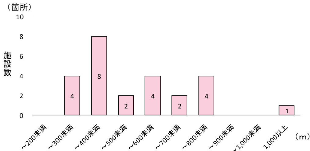
図-11 最も近い住宅までの風力発電施設からの距離
