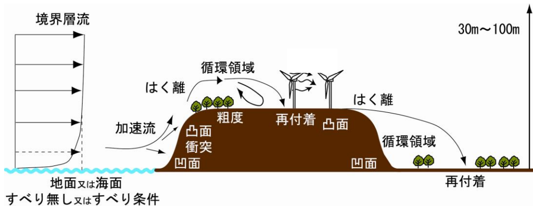
図 5-15 LAWEPS 工学モデルのモデリングで考慮された物理現象
