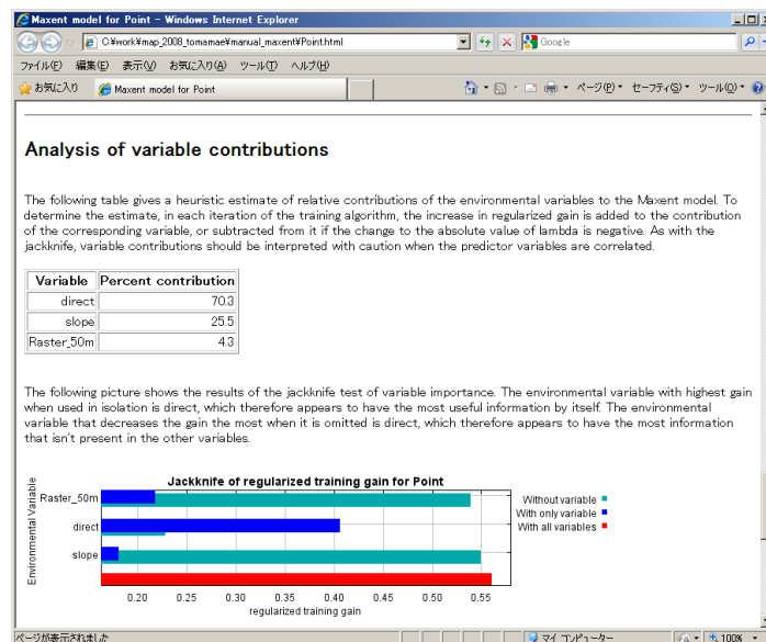
図 5-37 環境要因の寄与率
