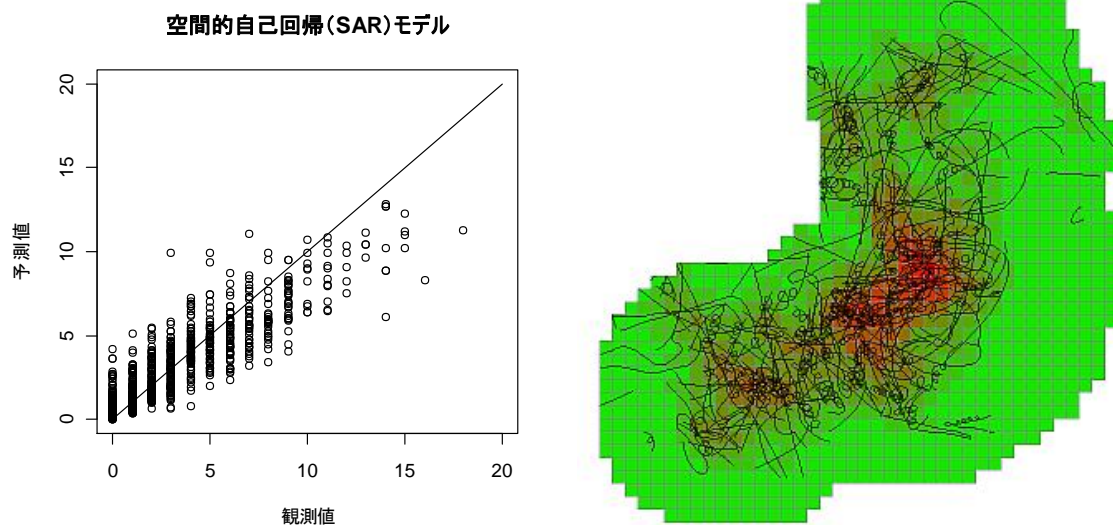
図 5-27 観測値と予測値の散布図(空間的自己回帰モデル)、およびポテンシャルマップ
