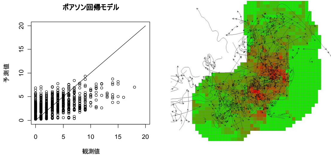
図 5-26 観測値と予測値の散布図(ポアソン回帰モデル)
