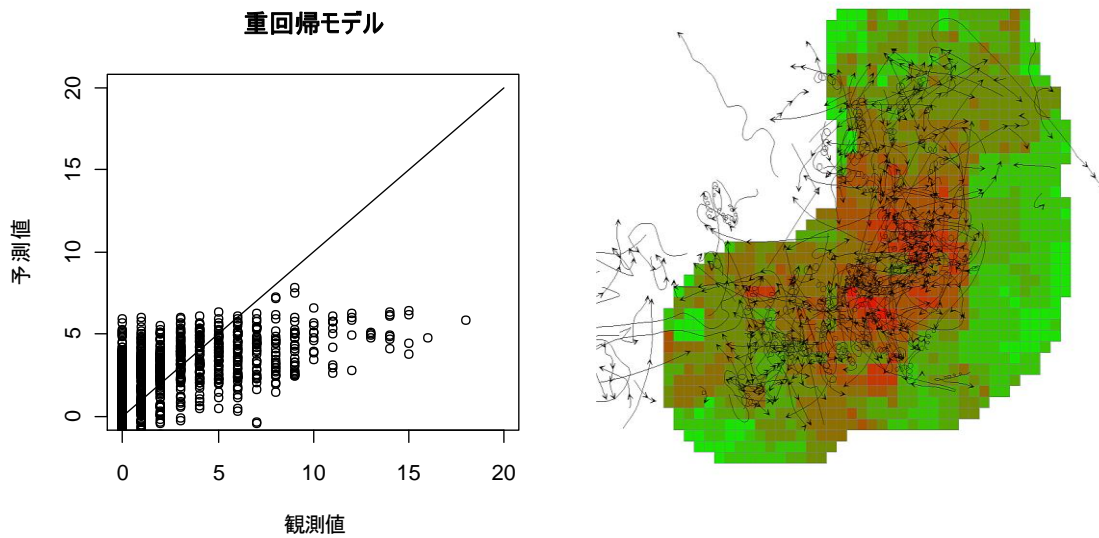
図 5-25 観測値と予測値の散布図(重回帰モデル)、およびポテンシャルマップ
