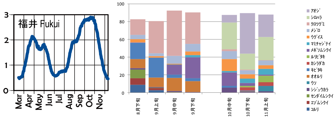
図 5- 7 ウインドプロファイラ(福井)の鳥エコーに基づく鳥類の通過頻度(左図)と織田山で標識された渡り鳥の種構成(右図)(左図縦軸は、10 分間の鳥エコー頻度の平均値である。鳥エコー頻度:0~11 までの値をとり、数が多いほど鳥が高頻度で通過することを示している)
