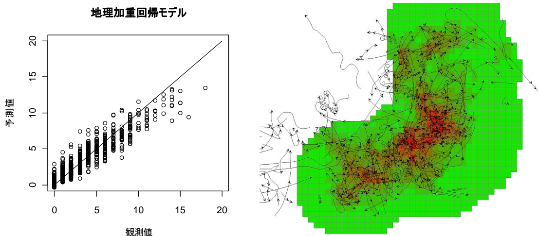
図 5-28 観測値と予測値の散布図(地理加重回帰モデル)、およびポテンシャルマップ
