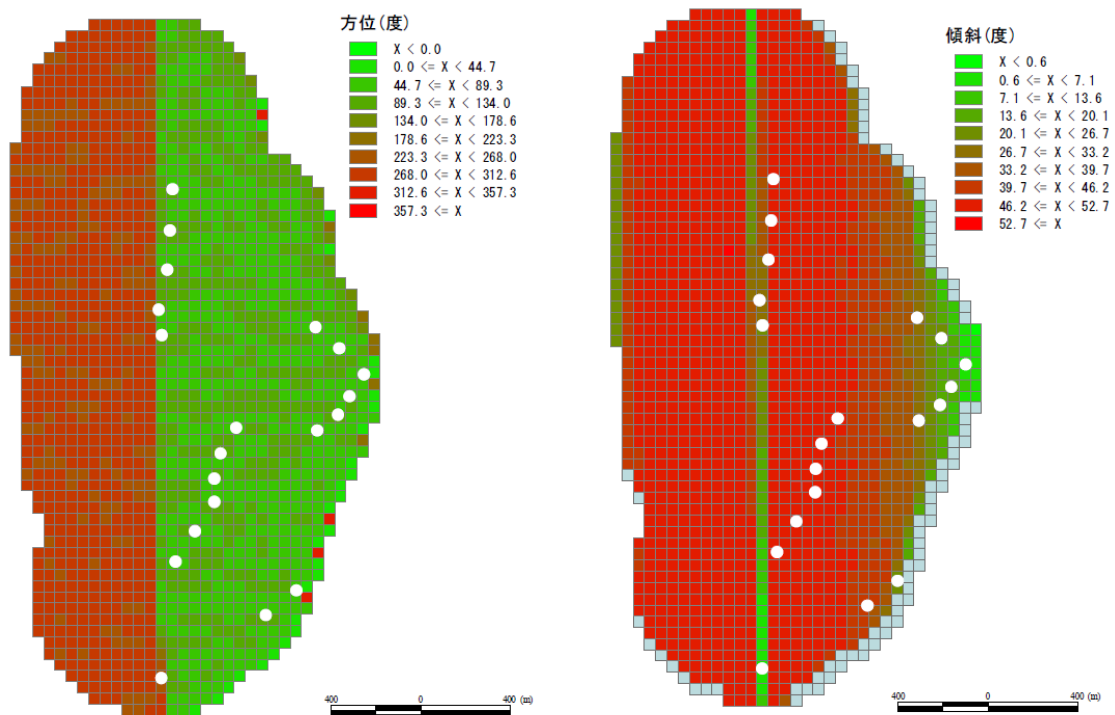
図 5- 35 前掲の標高値から斜面方位(左)と傾斜度(右)を作成
