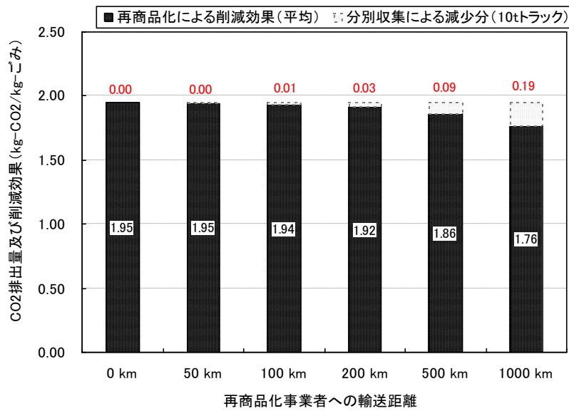
図 24 再商品化事業者への輸送距離別 CO2 削減効果（10t トラック；ごみ 1t あたり）
