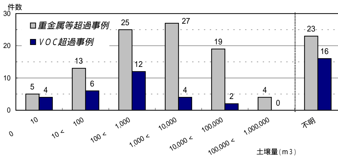
图4 污染土壤量
