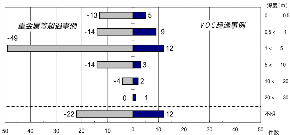
图2 污染深度
