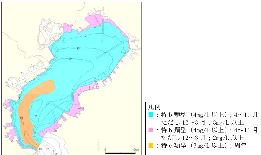
図 7 東京湾の底層 D0 の水域類型の当てはめ例 (目標設定種の全種を対象)
