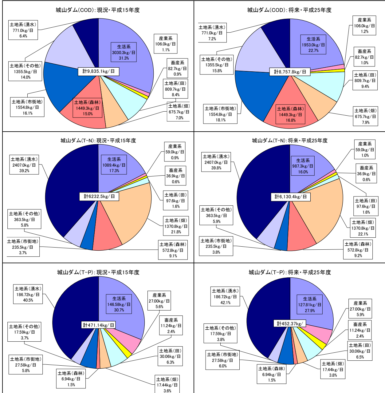
図 4. 19 城山ダム貯水池における現況と将来の汚濁負荷量比較
