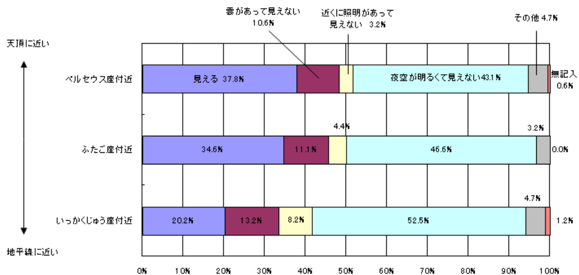
図3 肉眼による天の川の観察(冬期)
