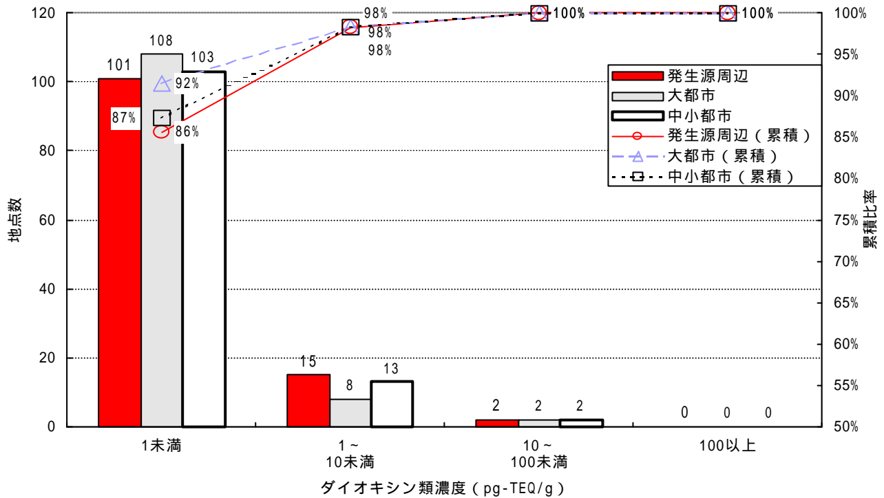
図2 地域別土壌中ダイオキシン類濃度の分布
