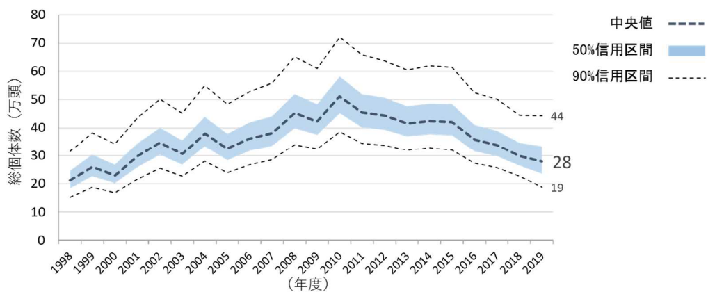
図 I-11 九州地方におけるイノシシの推定個体数の推移 (2020 (令和2) 年度実施)
