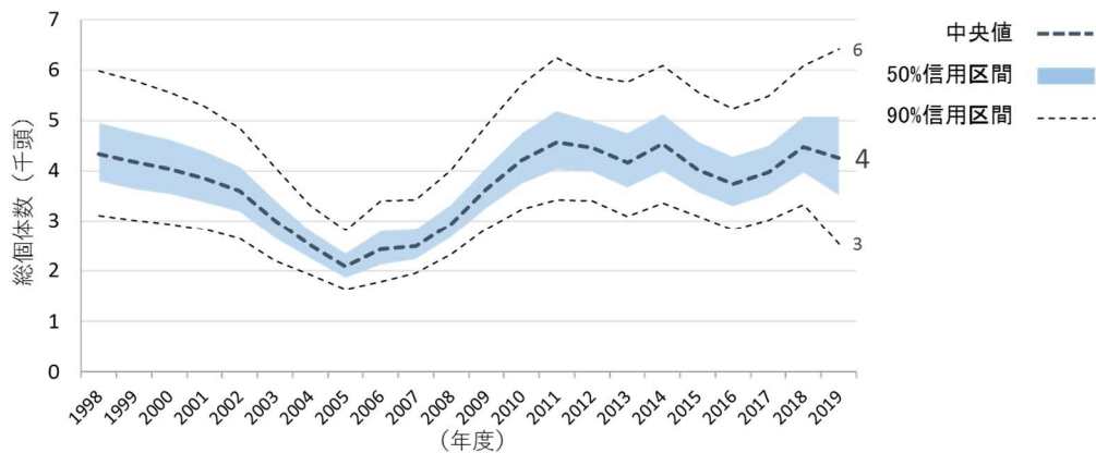
図 I-12 沖縄県におけるイノシシの推定個体数の推移 (2020 (令和2) 年度実施)
