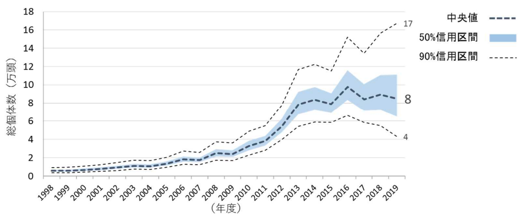
図 I-5 東北地方におけるイノシシの推定個体数の推移 (2020 (令和2) 年度実施)
