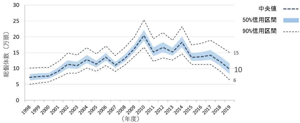
図 I-7 中部地方におけるイノシシの推定個体数の推移 (2020 (令和2) 年度実施)
