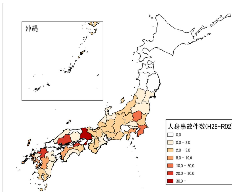
図 IV-5 イノシシによる人身事故件数（2016（平成 28）～2020（令和 2）年度）
