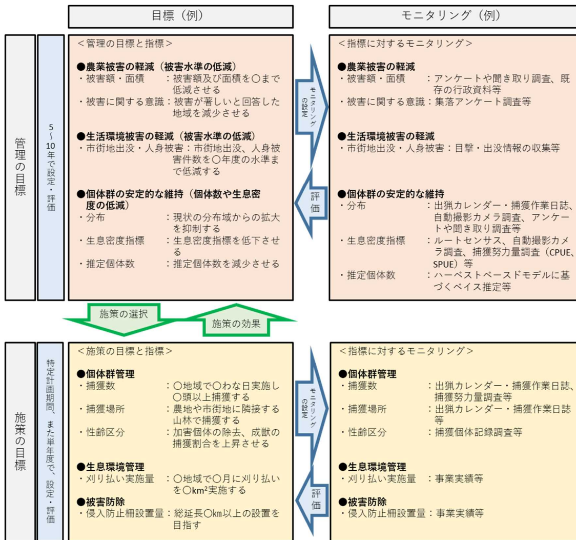
図 II-3 管理の目標と施策の目標、指標とモニタリングの対応例
