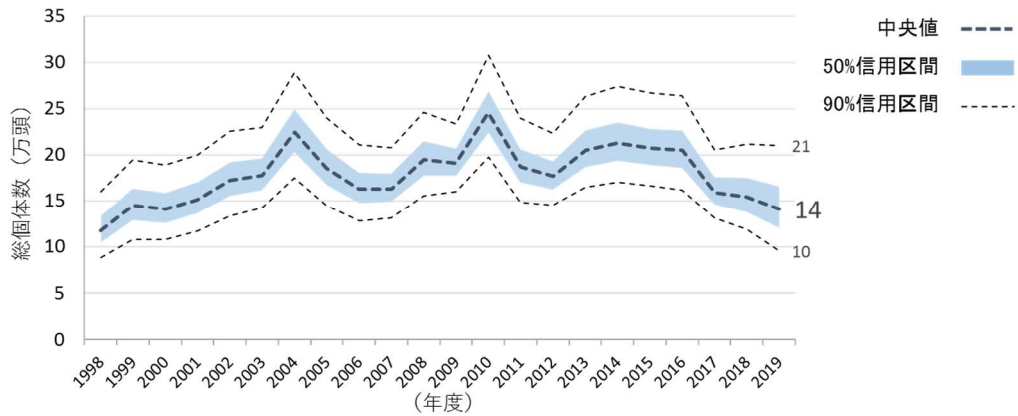
図 I-9 中国地方におけるイノシシの推定個体数の推移 (2020 (令和2) 年度実施)
