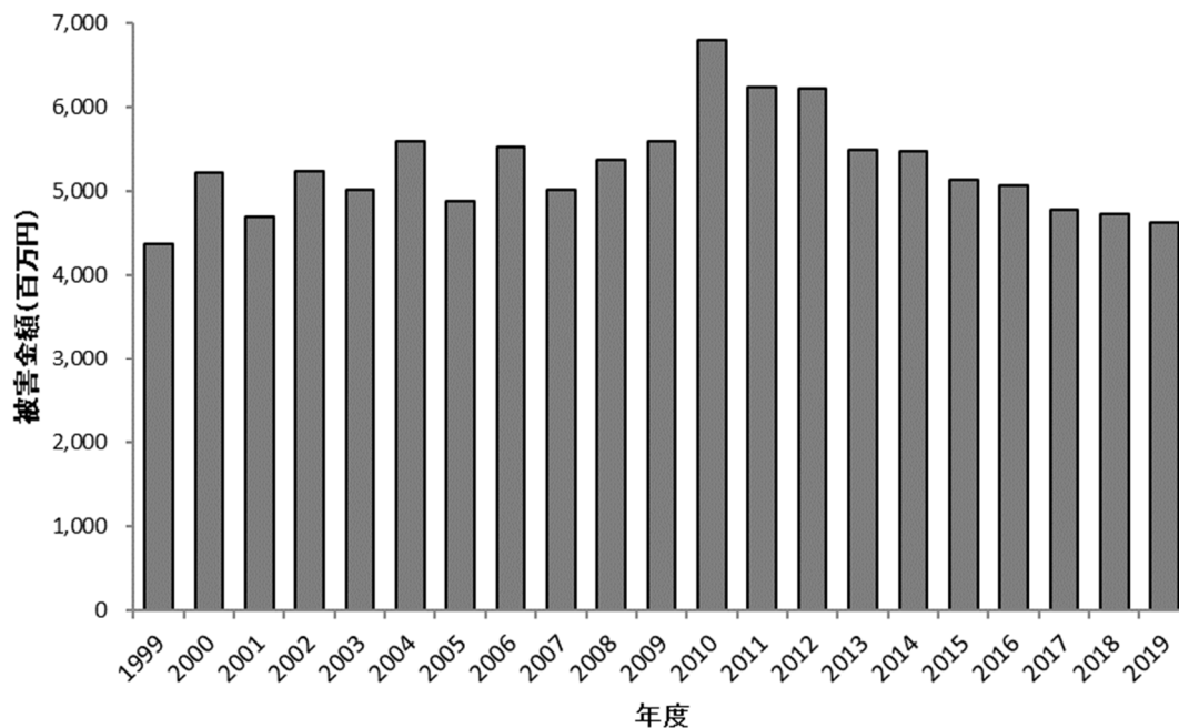
図 IV-2 イノシシによる農業被害金額の推移（百万円）
