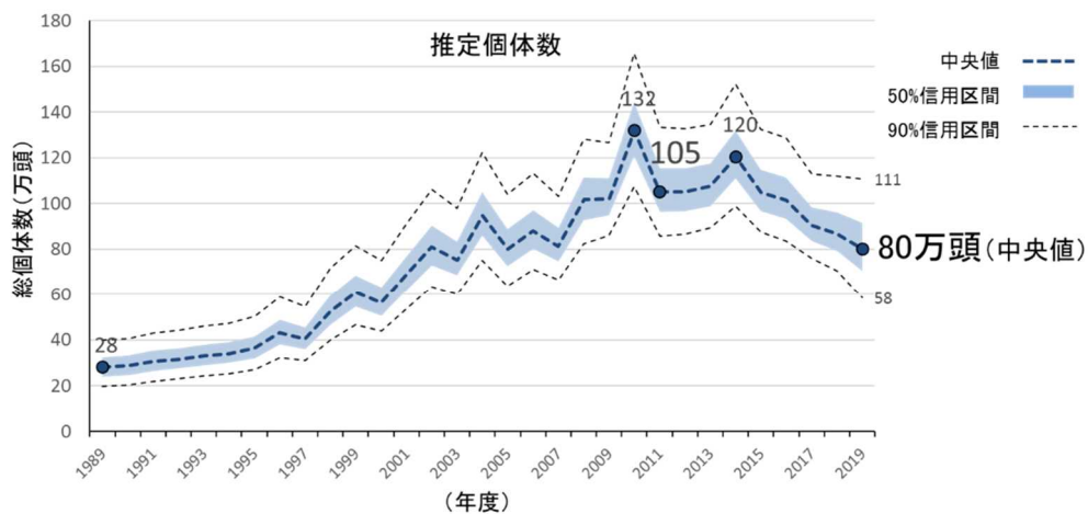
図 I-4 イノシシの推定個体数の推移 (2020 (令和2) 年度実施)
