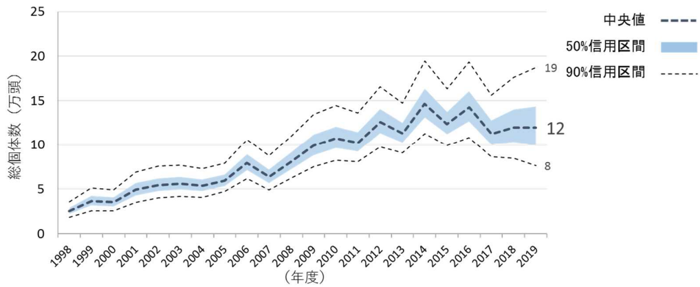
図 I-6 関東地方におけるイノシシの推定個体数の推移 (2020 (令和2) 年度実施)
