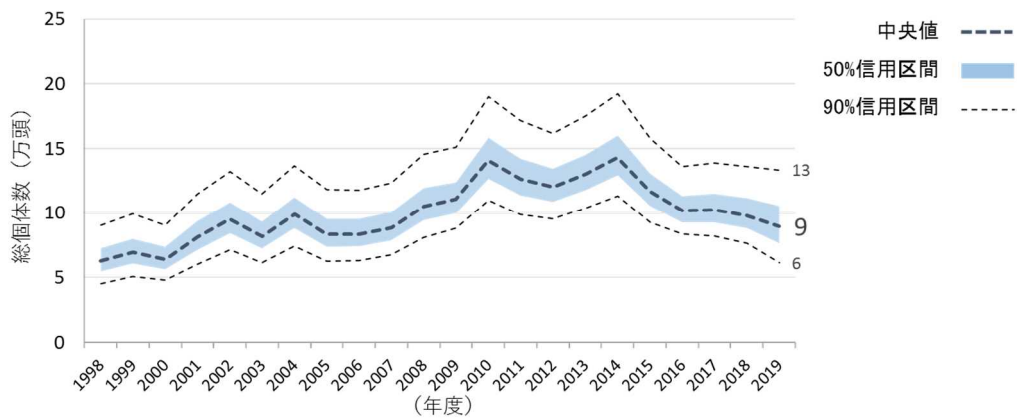
図 I-10 四国地方におけるイノシシの推定個体数の推移 (2020 (令和2) 年度実施)
