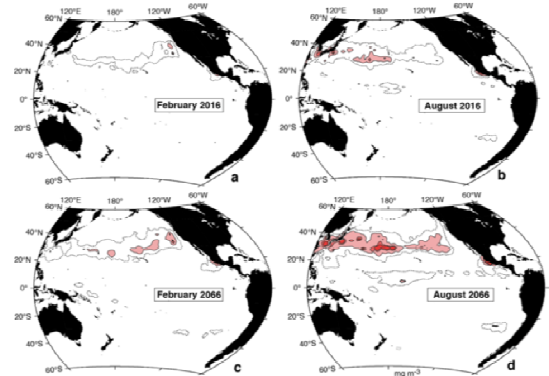
図 2016年現在と50年後の浮遊マイクロプラスチックの重量濃度分布シミュレーション(海水1m 3 あたりの浮遊重量) 左側は2月で右側は8月の分布を示す。最も濃い赤のトーンは1000 mg/m 3 以上の重量濃度を示す海域を表している。
