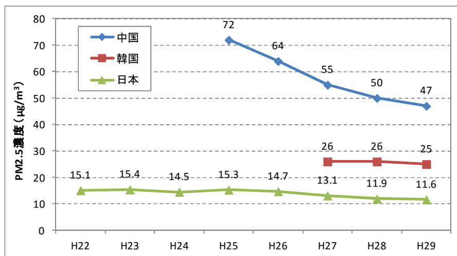
図 1-5 日中韓の PM2.5 濃度の年平均値の推移
