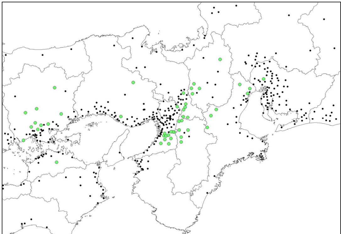
図2-6 平成29年度の注意報レベル(0.12ppm以上)の濃度が出現した日数の分布 (関東地域、関西地域：一般局)
