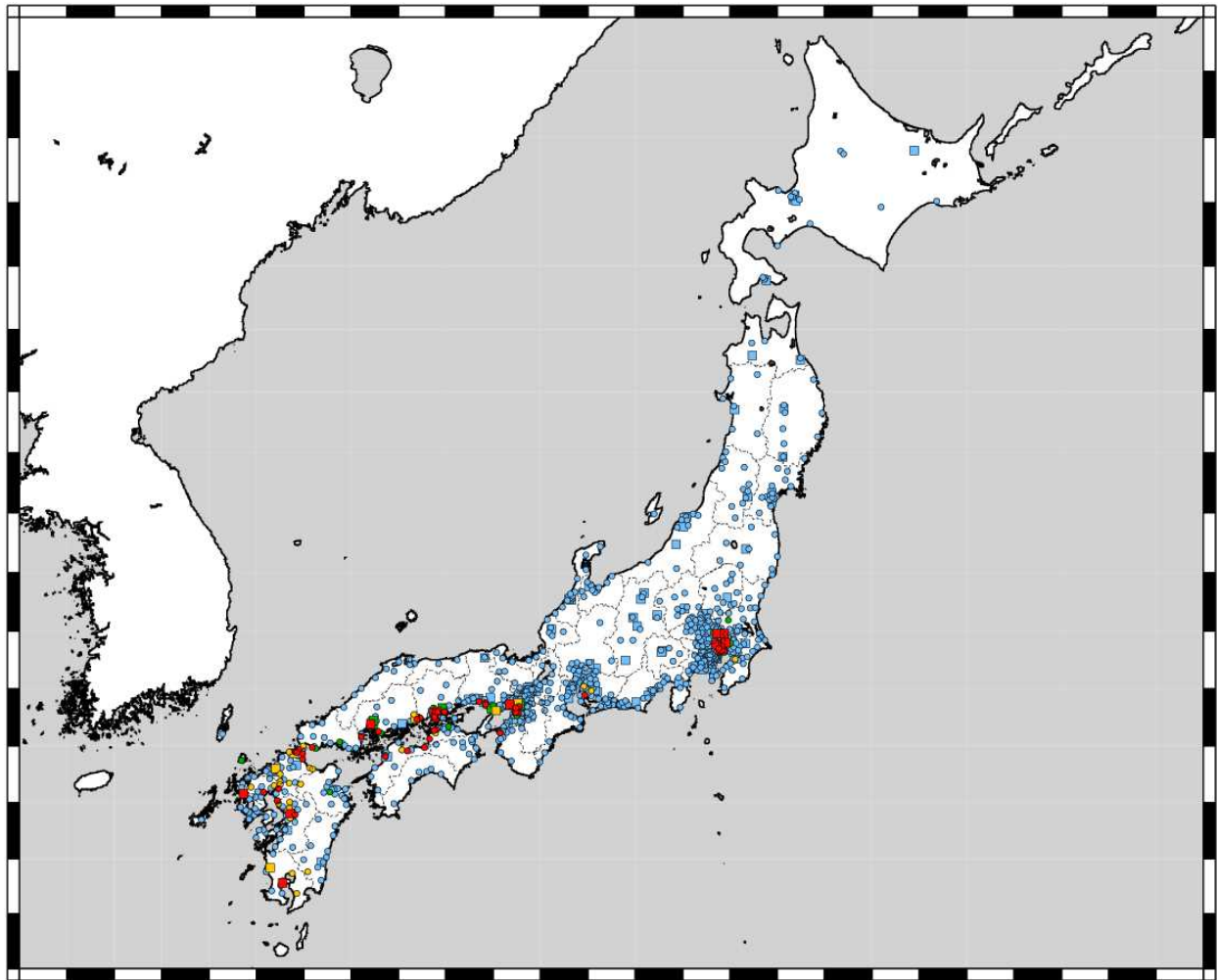
図 1-4-2 平成 29 年度の全国における PM2.5 環境基準達成状況 (○：一般局、□：自排局)
