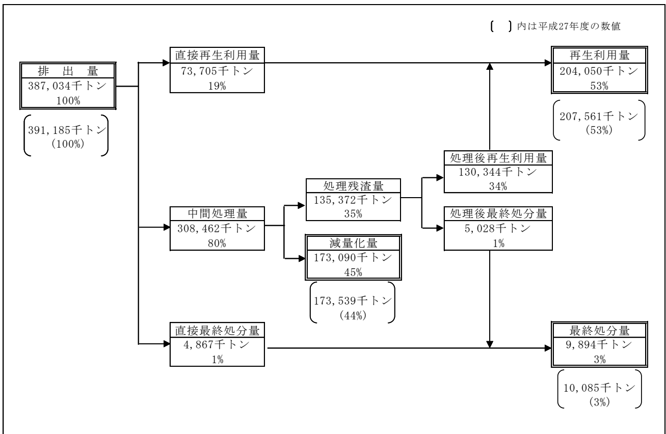
図 1-5 全国産業廃棄物の処理フロー（平成 28 年度実績）
