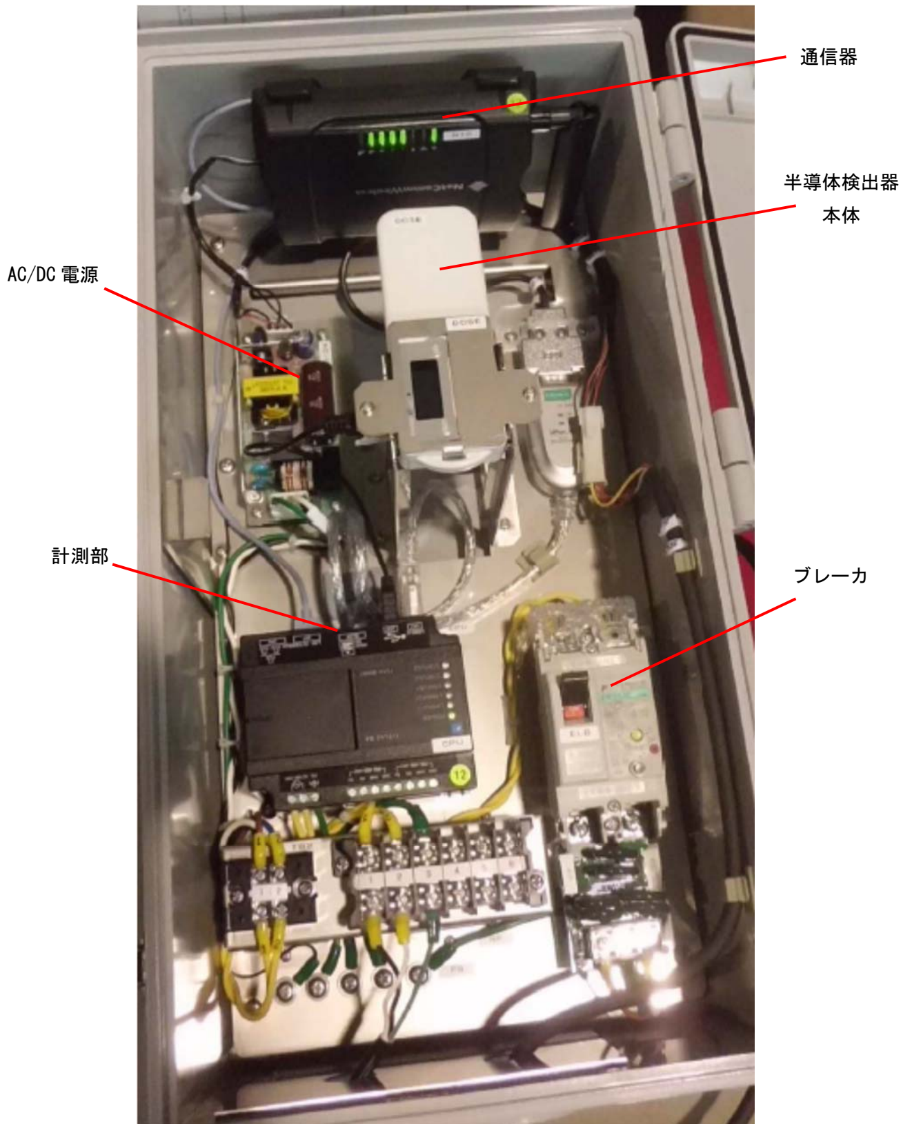
対策前のモニタリングポスト本体内部の機器構成
