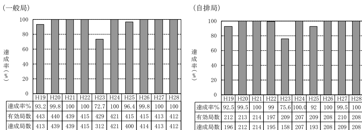
図2-4 自動車NOx・PM法の対策地域における浮遊粒子状物質の環境基準達成率の推移
