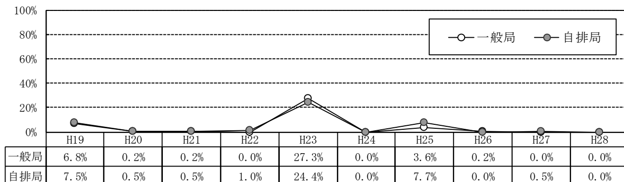
図2-5 自動車NOx・PM法の対策地域における環境基準を超える日が2日以上連続することにより非達成となった測定局の割合
