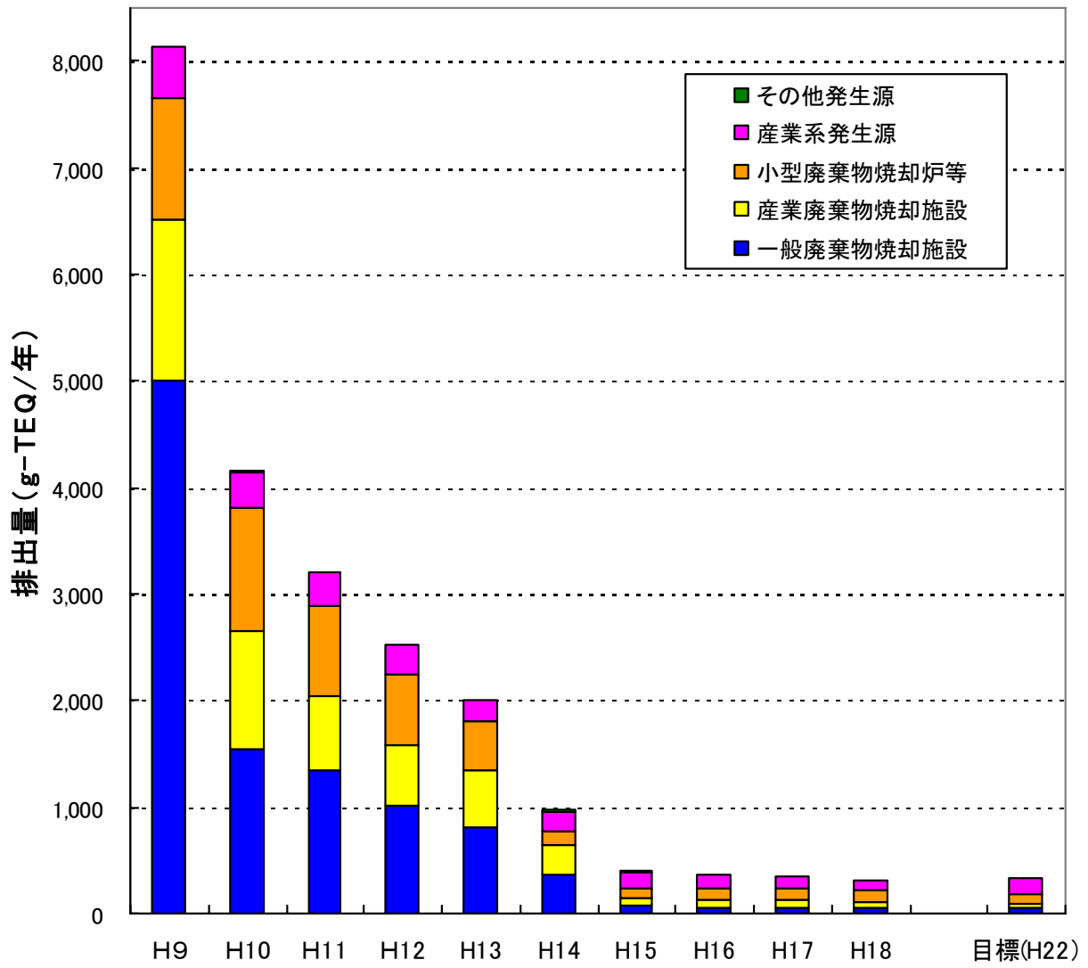
ダイオキシン類の排出総量の推移
