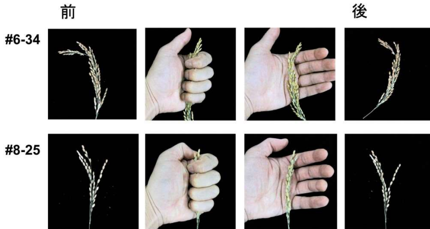
図4. 脱粒性
