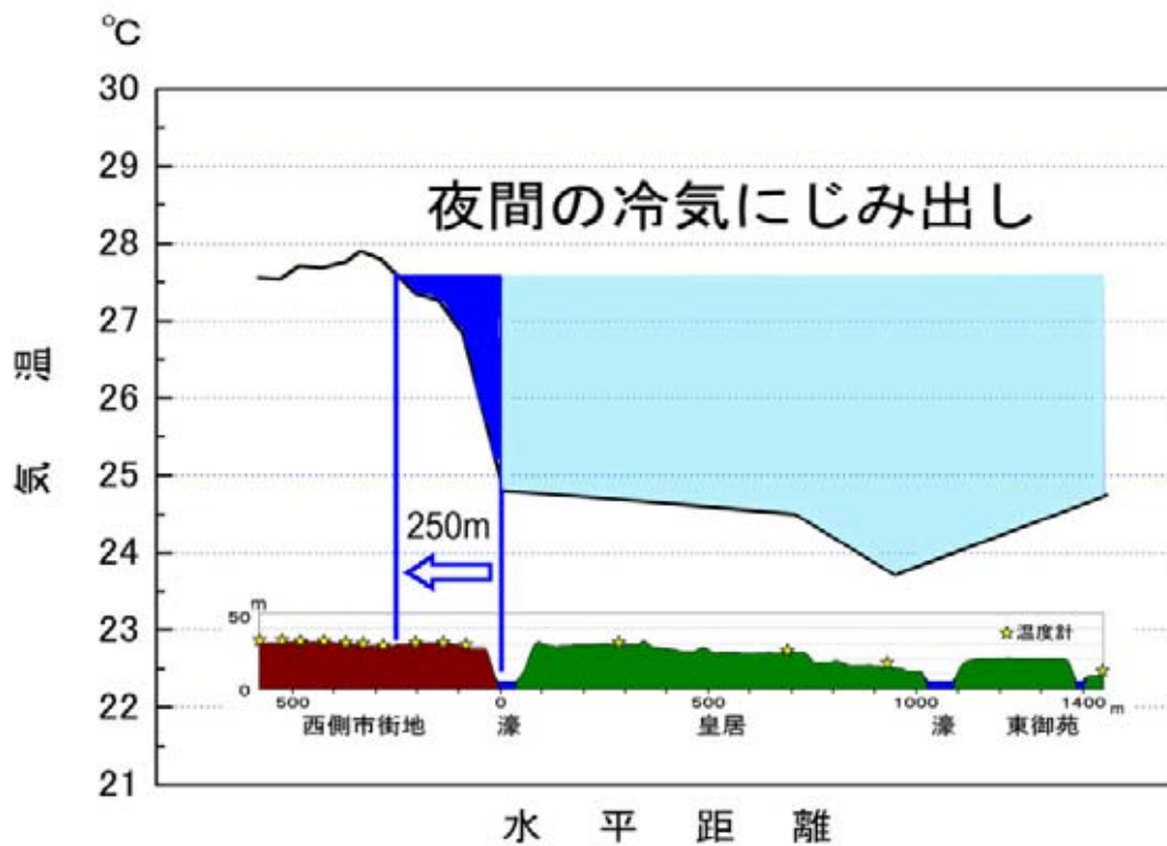
図5 冷気のにじみ出しの観測結果
