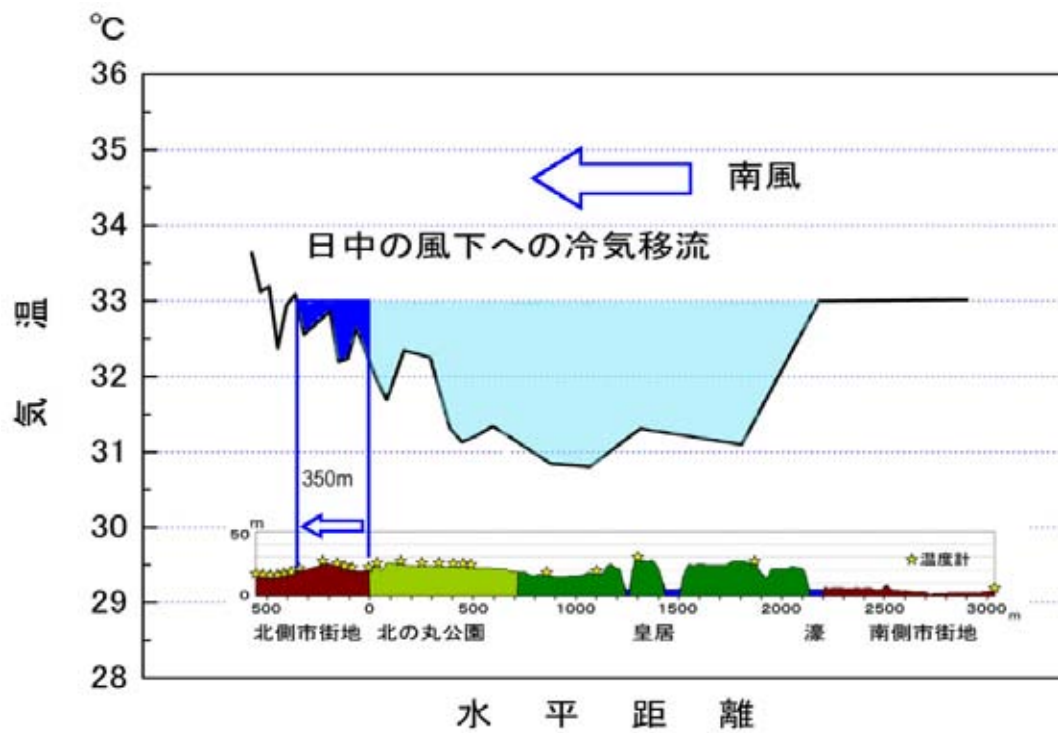
図4 冷気の移流の観測結果
