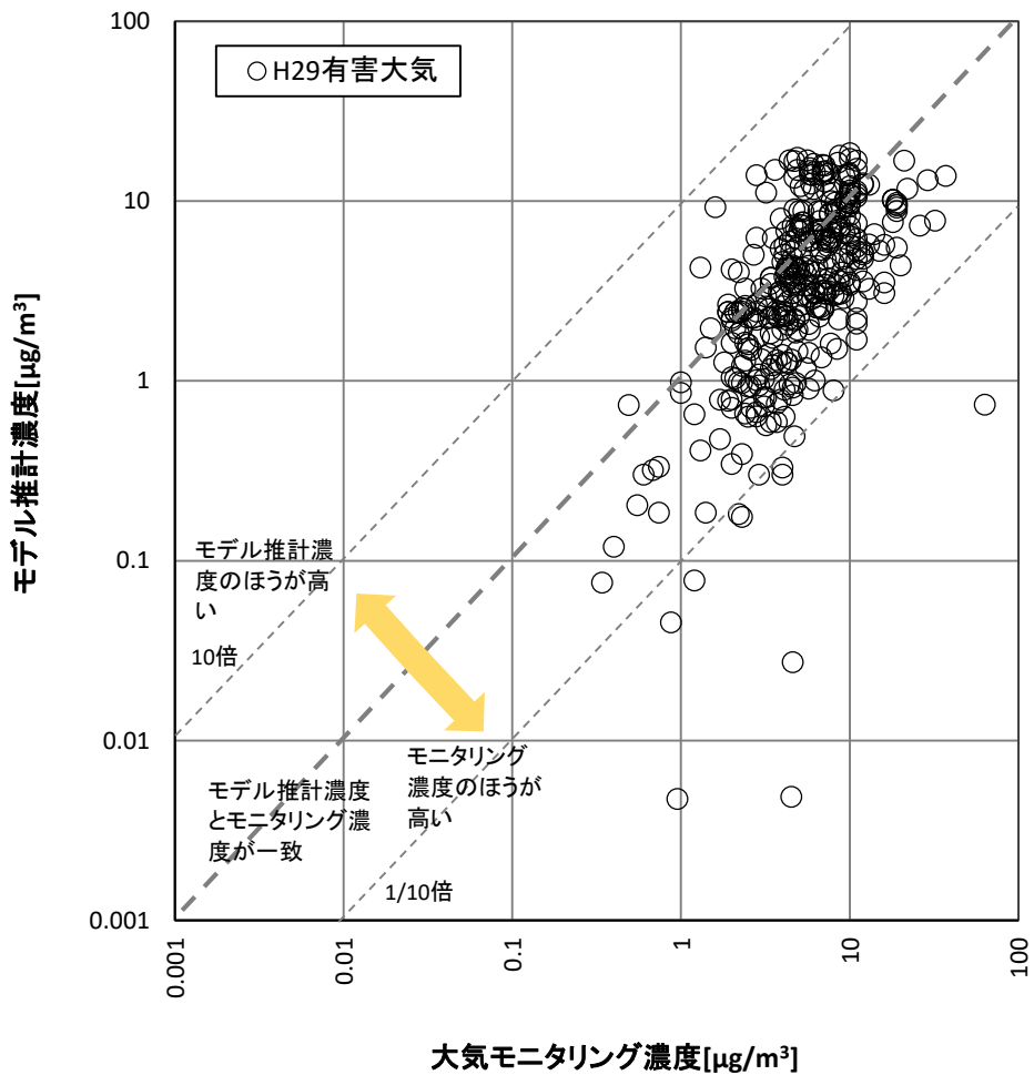
図 3 G-CIEMS 推計大気濃度 (PRTR 平成 29 年度実績) と 9 大気モニタリング濃度 (有害大気平成 29 年度) の比較
