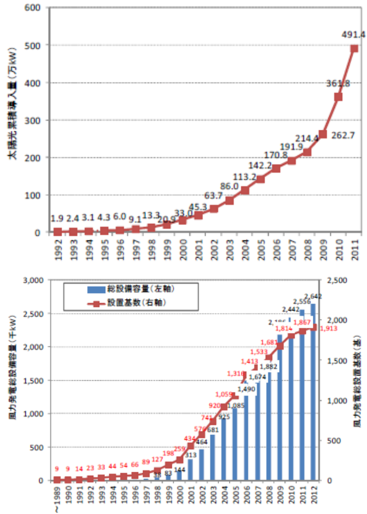
図 3-19 太陽光発電 (上) および風力発電 (下) の導入量
