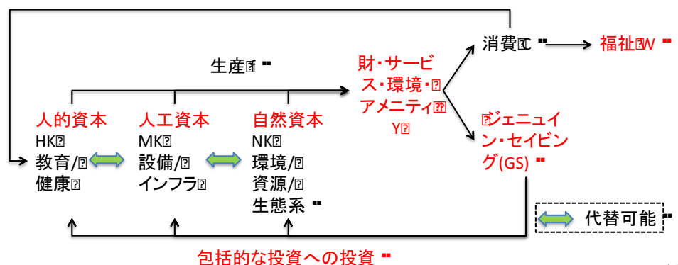
図 3.1 GDP と GS
