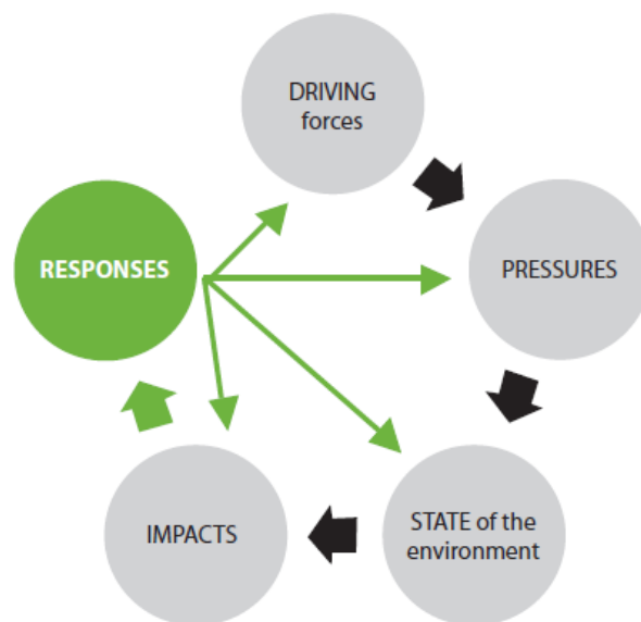
図 2.6 DPSIR 枠組み
