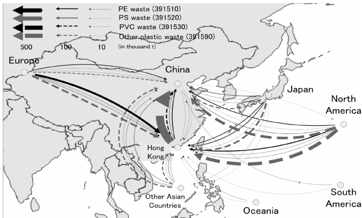
図 . プラスチック廃棄物の越境異動の状況
