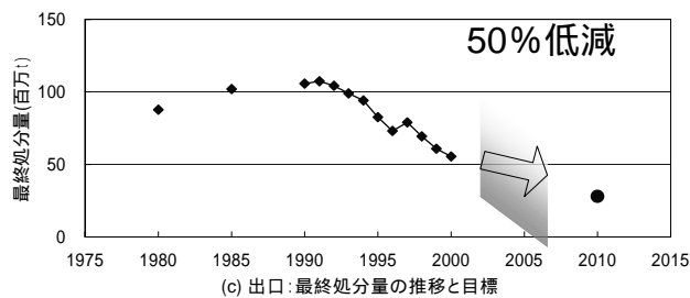
循環基本計画の3つの物質フロー指標の推移と数値目標
