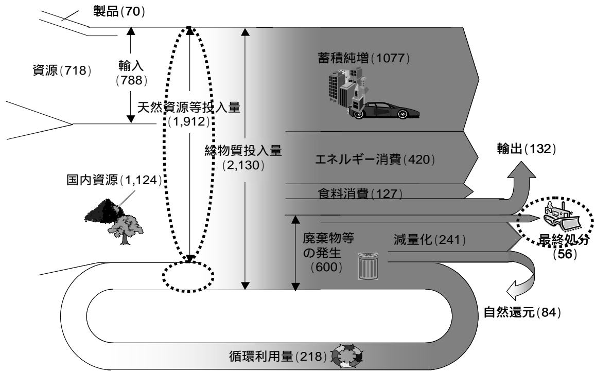
平成12年度の我が国における物質フローの模式図（環境省作成）
