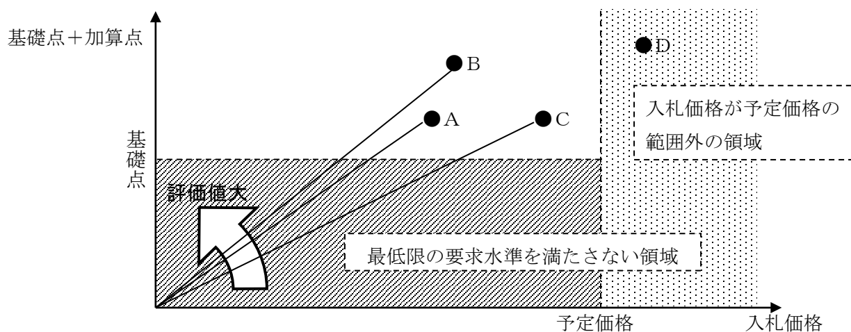
図V-3-4 除算方式のイメージ
