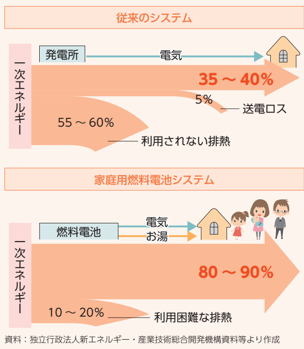
図3-1-11 従来の商用電力と家庭用コージェネレーションシステムとのエネルギー利用率比較
