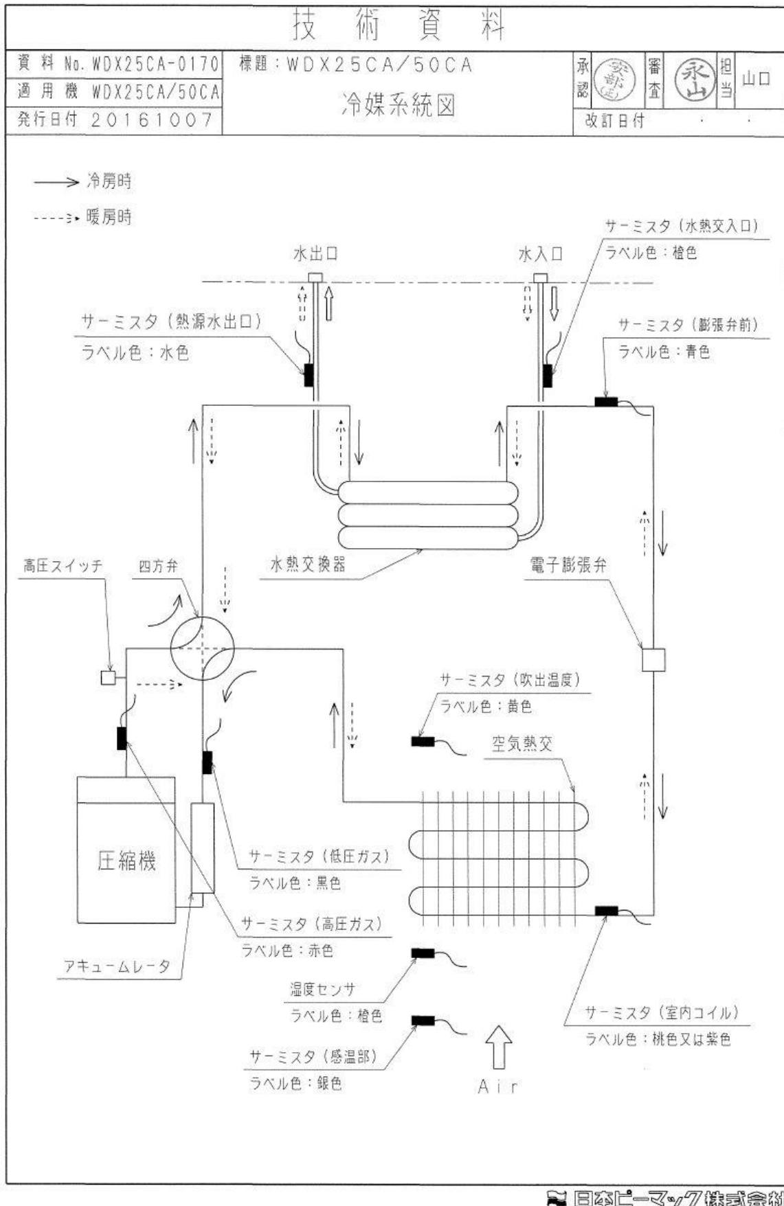
図 3-3 実証対象技術の構造 (冷媒系統図)
