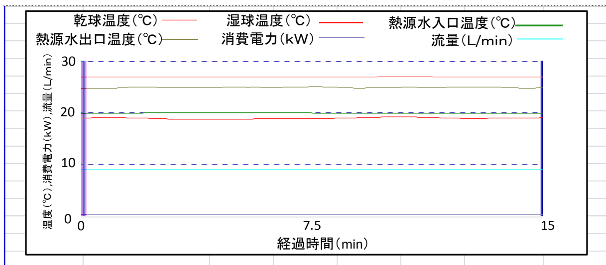
図 6-3 各水温の安定確認
