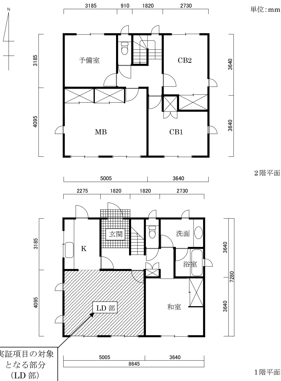
図 4-1 計算用住宅モデル（平面図）
