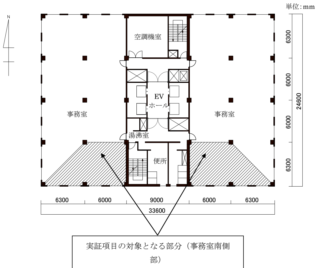
図 4-2 計算用オフィスモデル（平面図）
