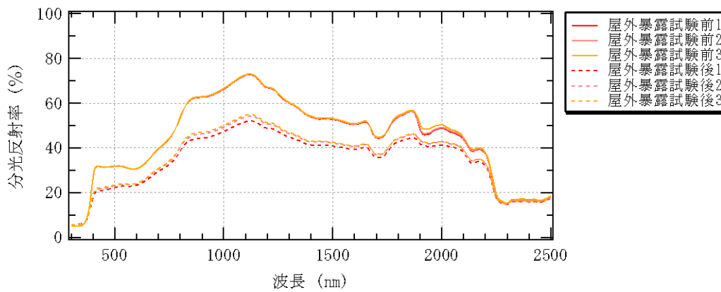
図 5-3 分光反射率測定結果(N6)
