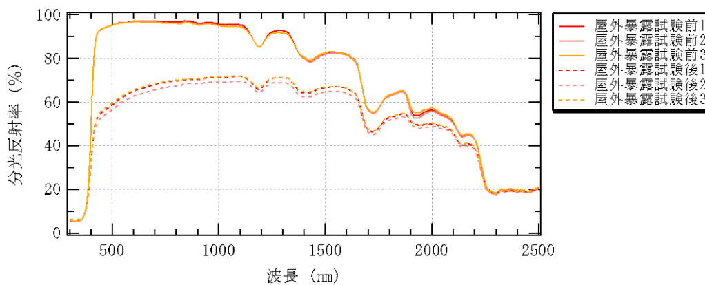
図 5-4 分光反射率測定結果(トゥルーホワイト)
