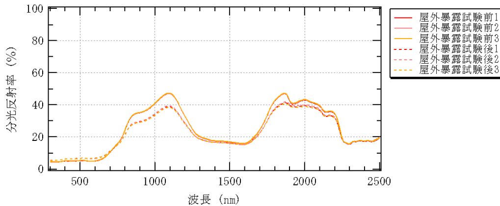
図 5-2 分光反射率測定結果(チャコール)
