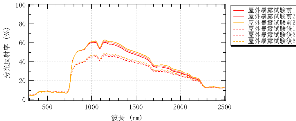
図 5-2 分光反射率測定結果 (ダークグレー)
