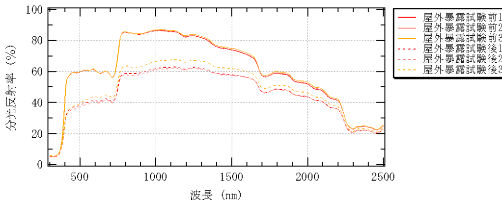
図 5-3 分光反射率測定結果 (ホワイトグレー)
