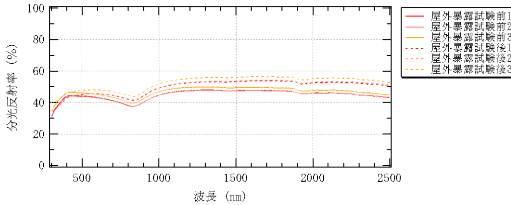
図 5-2 分光反射率測定結果 (シルバー)
