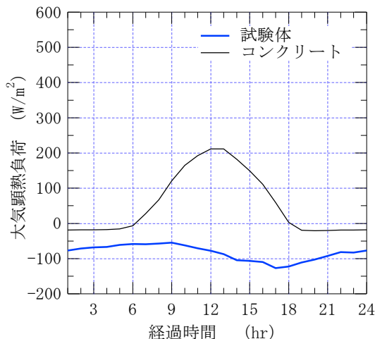
図 3-2 顕熱負荷の経時変化（地域：東京）
