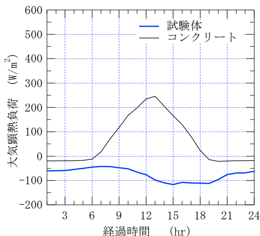
図 3-4 顕熱負荷の経時変化（地域：大阪）
