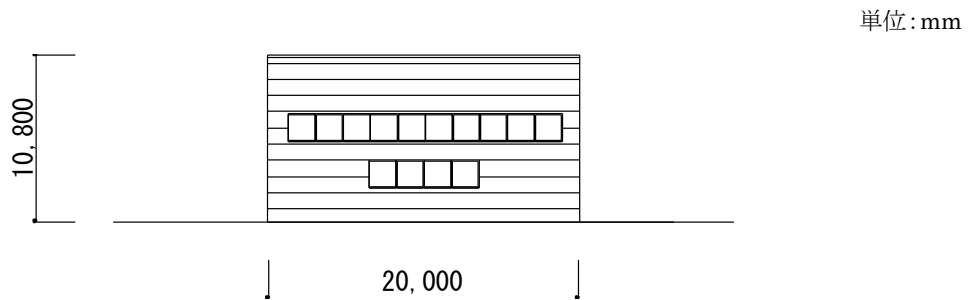
付図 2 計算用工場モデル（東側立面図）
