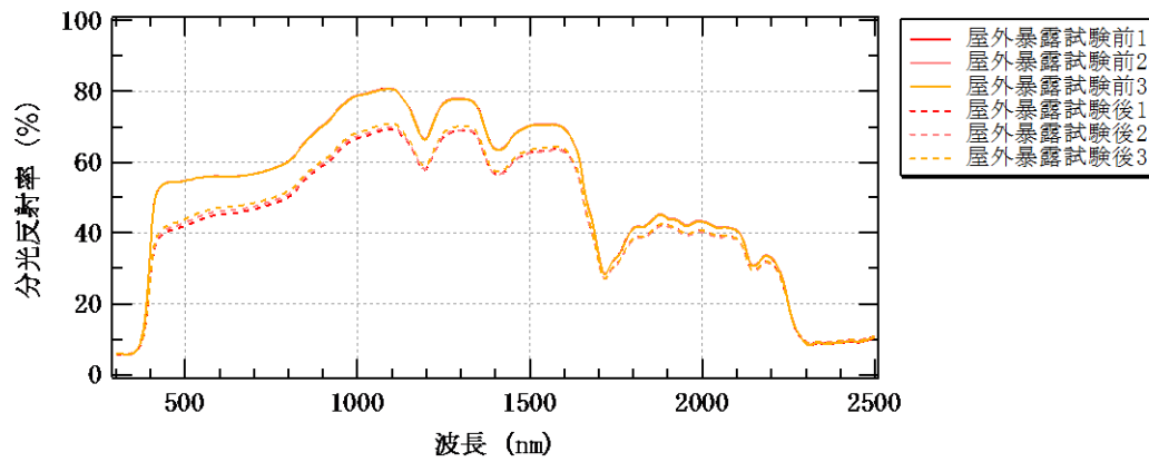
図 5-2 分光反射率測定結果
