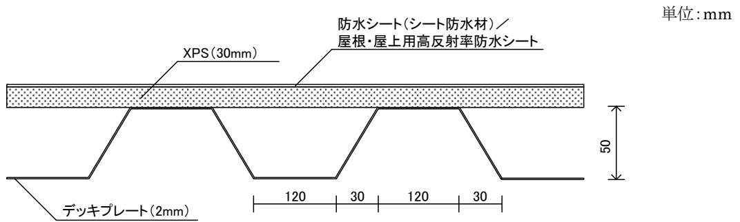
付図 3 屋根の形状（断面）
