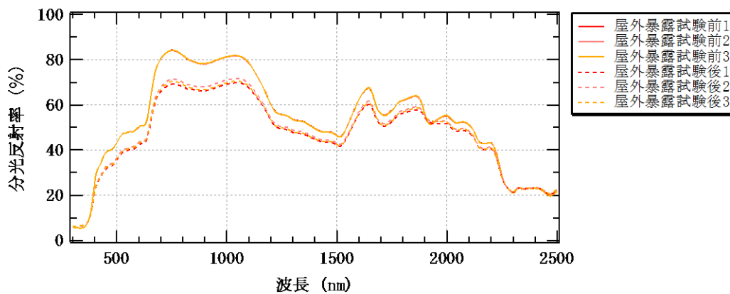
図 5-3 分光反射率測定結果 (遮熱ベージュ)
