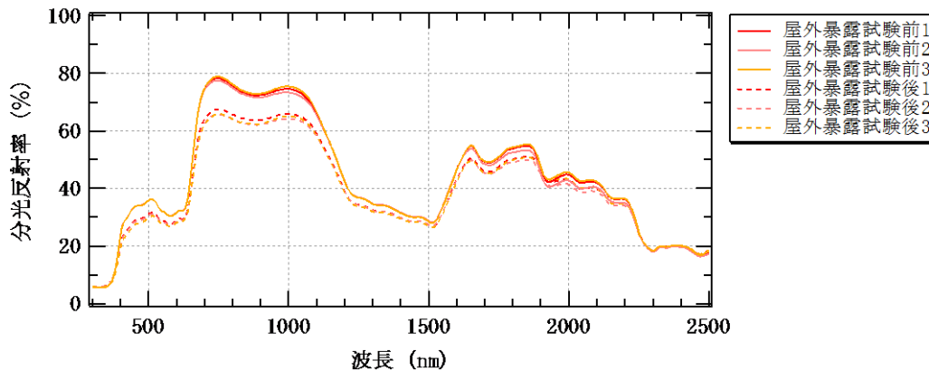
図 5-2 分光反射率測定結果 (遮熱グレー(N6))
