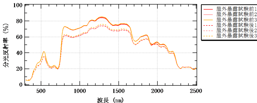
図 5-4 分光反射率測定結果 (遮熱グリーン)
