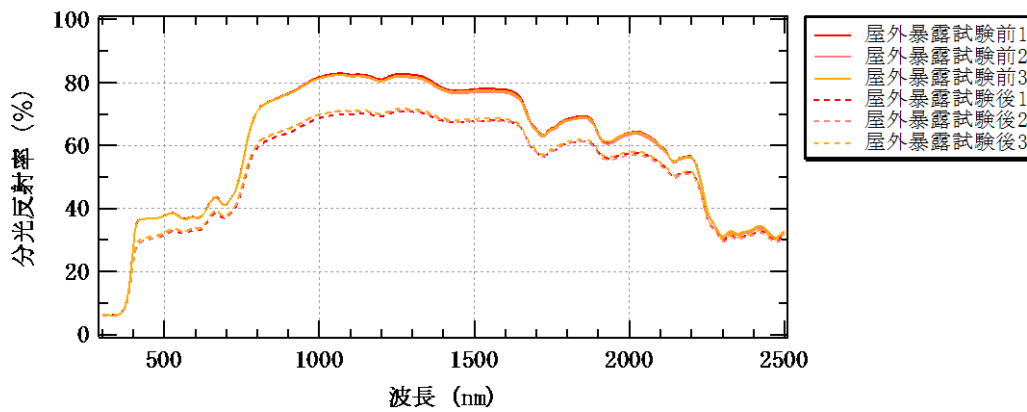
図-4 分光反射率測定結果(シルバーグレー)
