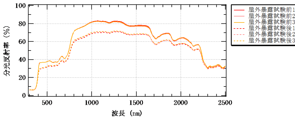
図 5-3 分光反射率測定結果(シルバーグレー)
