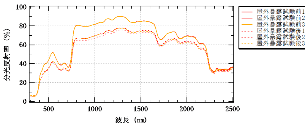
図 5-3 分光反射率測定結果(ライトグリーン)
