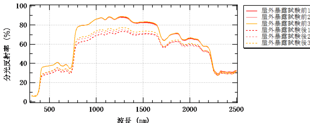
図 5-2 分光反射率測定結果(ライトグレー)
