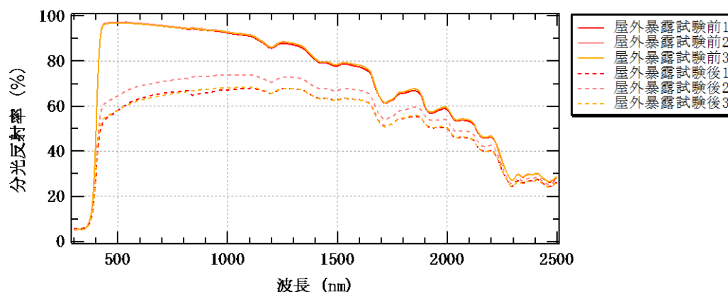
図 5-3 分光反射率測定結果（白色）
