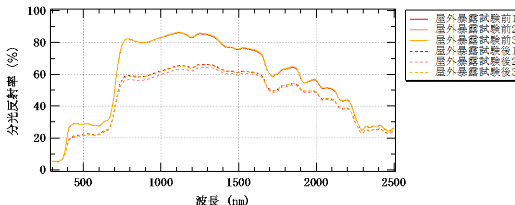
図 5-2 分光反射率測定結果（灰色）
