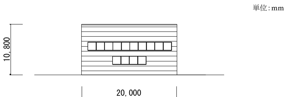
付図 2 計算用工場モデル（東側立面図）
