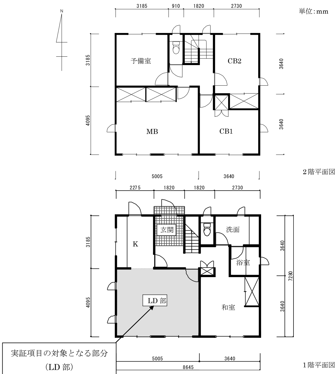
図 4-2 計算用住宅モデル（平面図）
