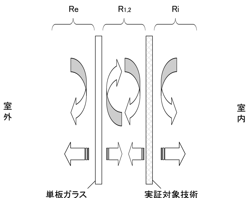
図 4-1 熱抵抗及び表面熱伝達抵抗の設定イメージ
